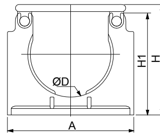
NFH-56 / 70 / 95
